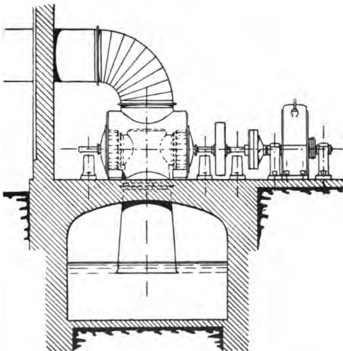
Fig. 37. Liegende Zwillingssturbinen mit Druckrohr.
